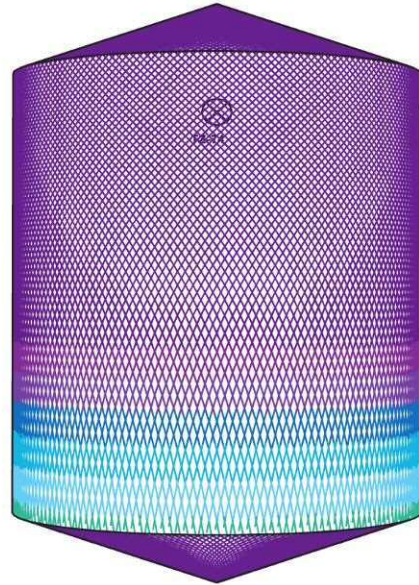
D5m H6m, Toftejorg TZ-74 自己洗浄型、4 x ø7 mm, 0% 時間 = 15.3 分、水消費量 = 4853 l
