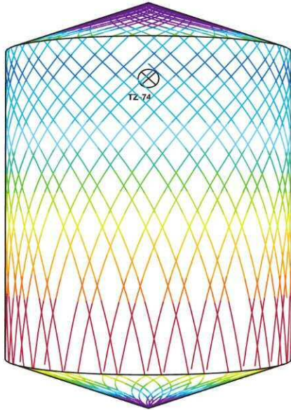
D5m H6m, Toftejorg TZ-74 自己洗浄型、4 x ø7 mm, 0% 時間 = 3.8 分、水消費量 = 1192 l
