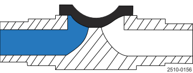
図 8. デルタ P 100%
