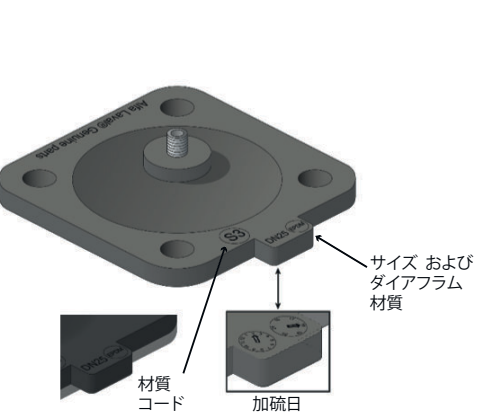
Alfa Laval EPDM Diaphragm
