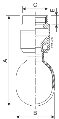
図 1. ネジ径
