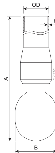
図 3. 溶接式
