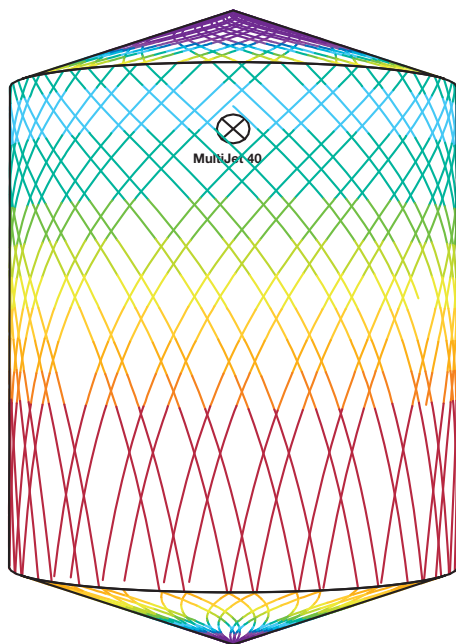
D5m H6m、Toftejorg MultiJet40、4 x ø6 mm、100% 時間 = 4.3 分、水消費量 = 887 l
