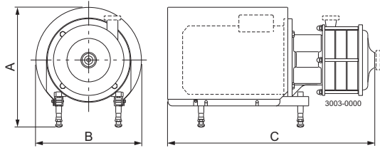
寸法 (mm)mm
