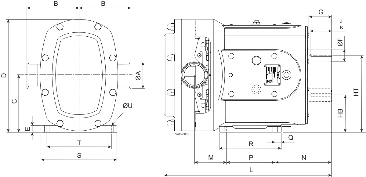
図 1. 水平ポート
