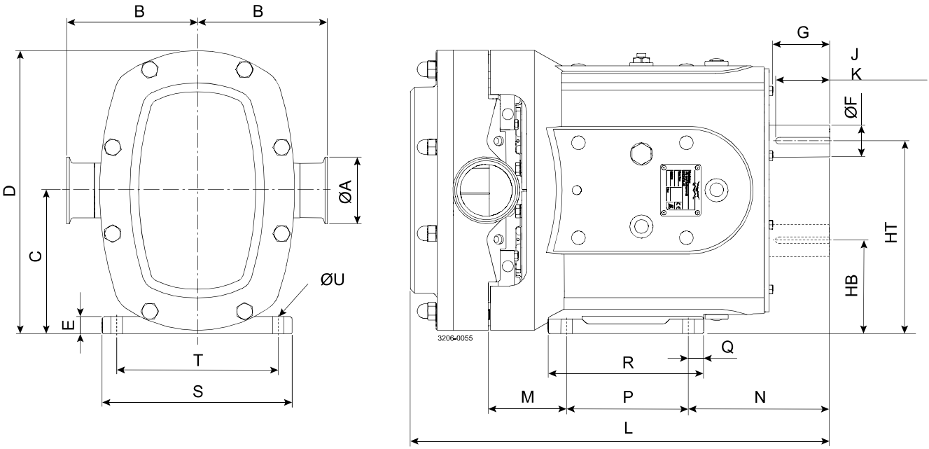
図 1. 水平ポート
