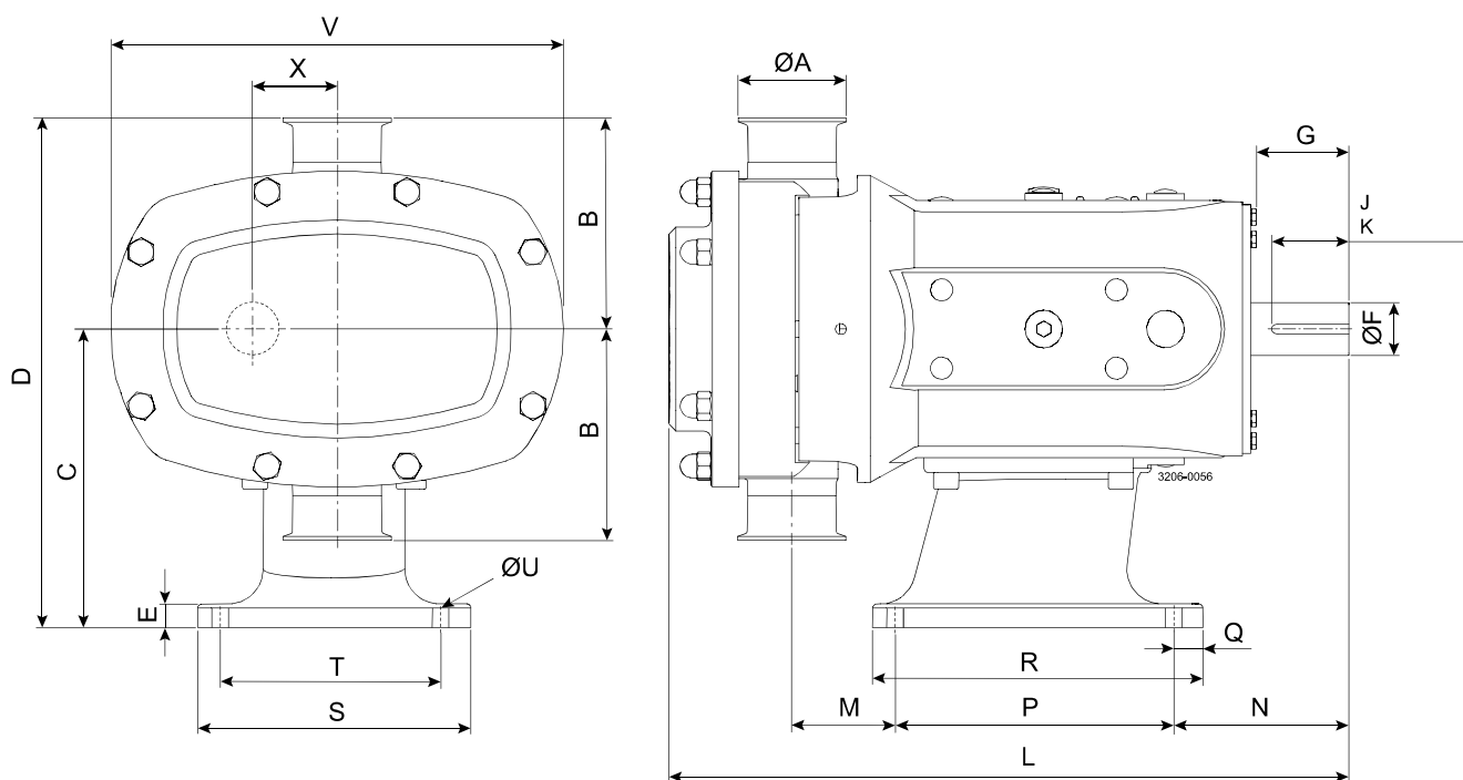
図 2. 垂直ポート
