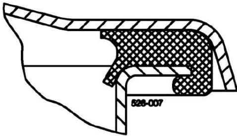
図2 - ダブルリップシールの構造断面
