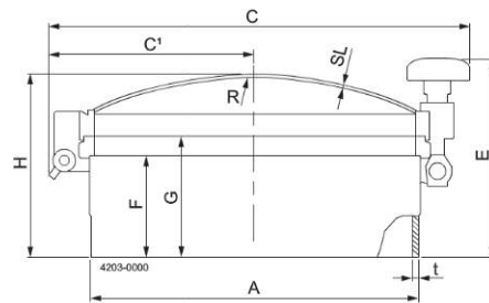
Fig. 2. Dimensions
